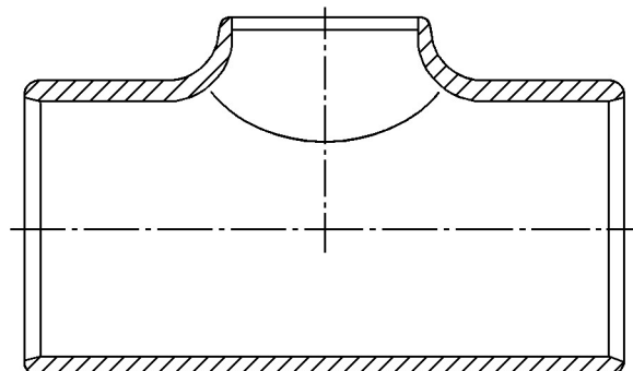
Reduceret T-stykke
