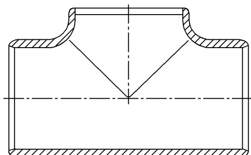
Lige T-stykke
